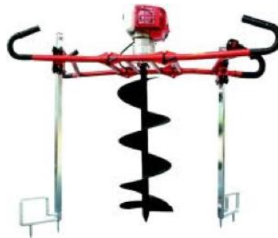
Image 6 : Tarière thermique à 2 hommes
