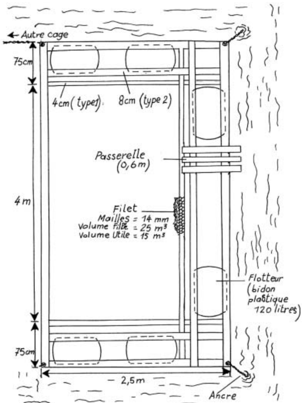
Figure 8.1 : Cage ivoirienne
