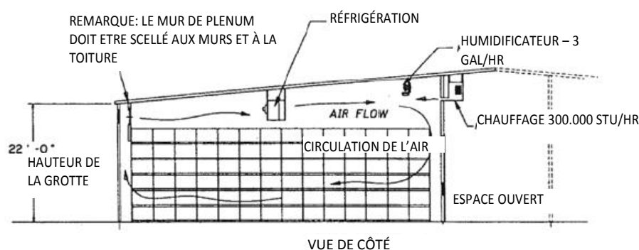
Vue de côté d'un diagramme de construction pour une ventilation horizontale négative
